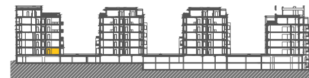
SCHÉMA PODLAŽÍ 1.NP
